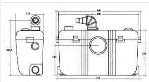
SANIBEST 2 wc+lavabo+ducha+lavadora
