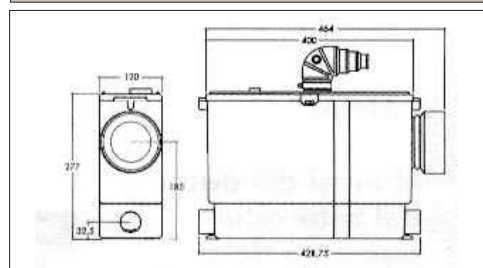
SANIPACK Wc suspendido+lavabo+ducha
