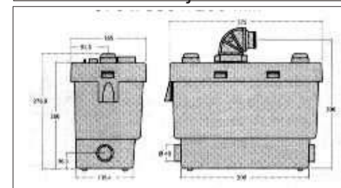
SANIVITE aguas usadas+lavadora+ lavavajillas
