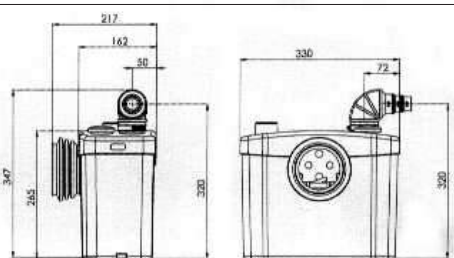
SANITOP wc+lavabo
