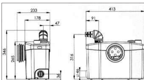
SANIPRO wc+lavabo+ducha
