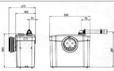
SANITRIT WC
